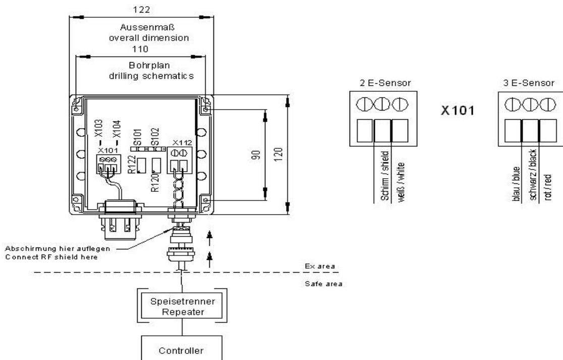
Image 2 / Picture 2: Têtes de détection pour gaz toxiques et oxygène / Sensor heads for toxic gases and oxygen
