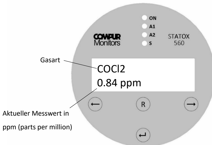
Abbildung 8: Stattox 560 Frontansicht
