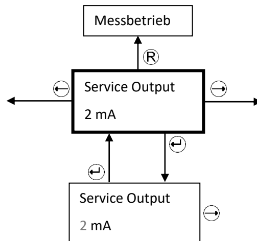
Abbildung 29: Ablaufdiagramm Service Output
