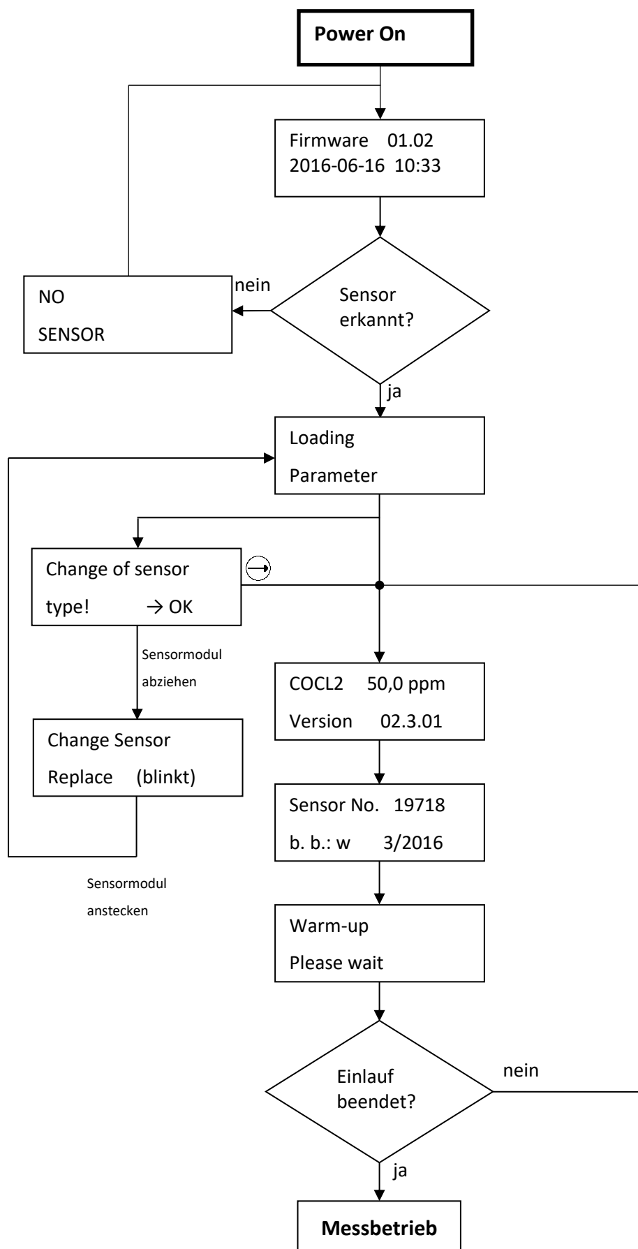
Abbildung 11: Ablaufdiagramm Einlaufphase
