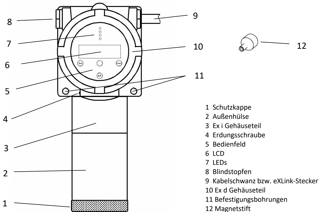
Abbildung 1: Messkopf Stattox 560
