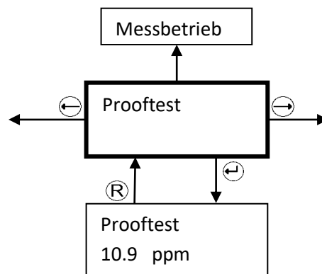
Abbildung 13: Ablaufdiagramm Prooftest
