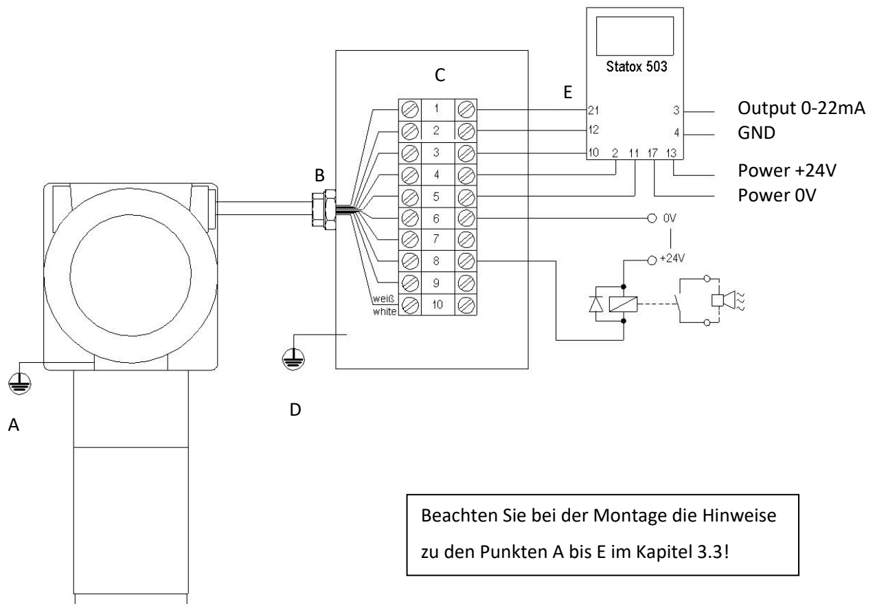
Abbildung 6: Anschlussschema des Statox 560 über ein Statox 503 Control Modul
